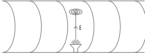
شكل ٣-١: يُجري رائد الفضاء تجربة يوجه فيها نبضة من الضوء نحو هدفها؛ بحيث ينتقل الضوء في اتجاه عمودي على اتجاه حركة المركبة.
